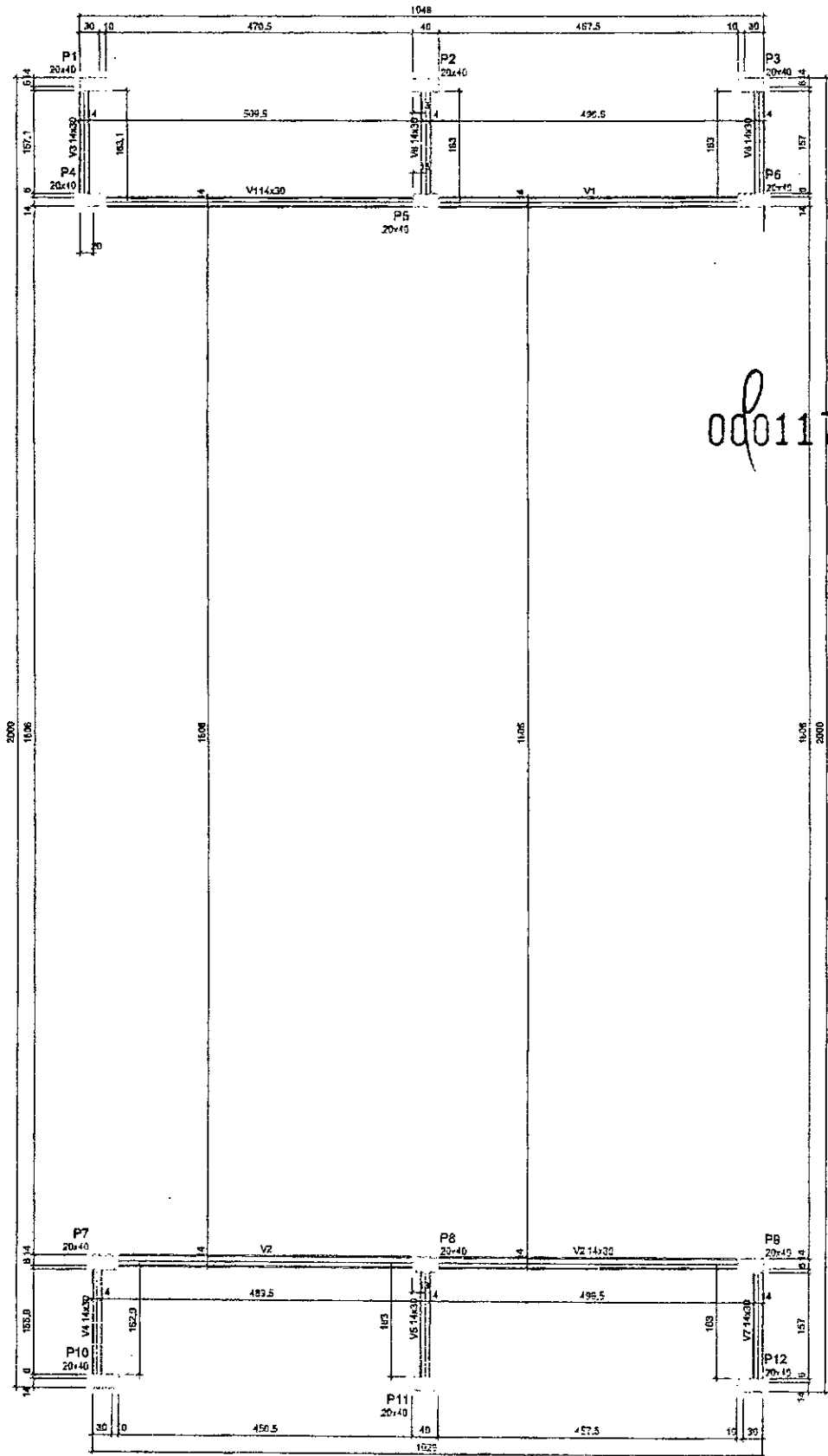
Forma do pavimento BALDRAME (Nível 0)
